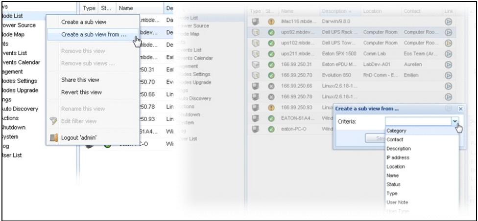
图 34. 子视图选择
